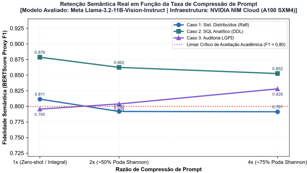
Figura 10.3 – Curva de retenção semântica (BERTScore F1) em função da razão de compressão e limiar de aceitação
